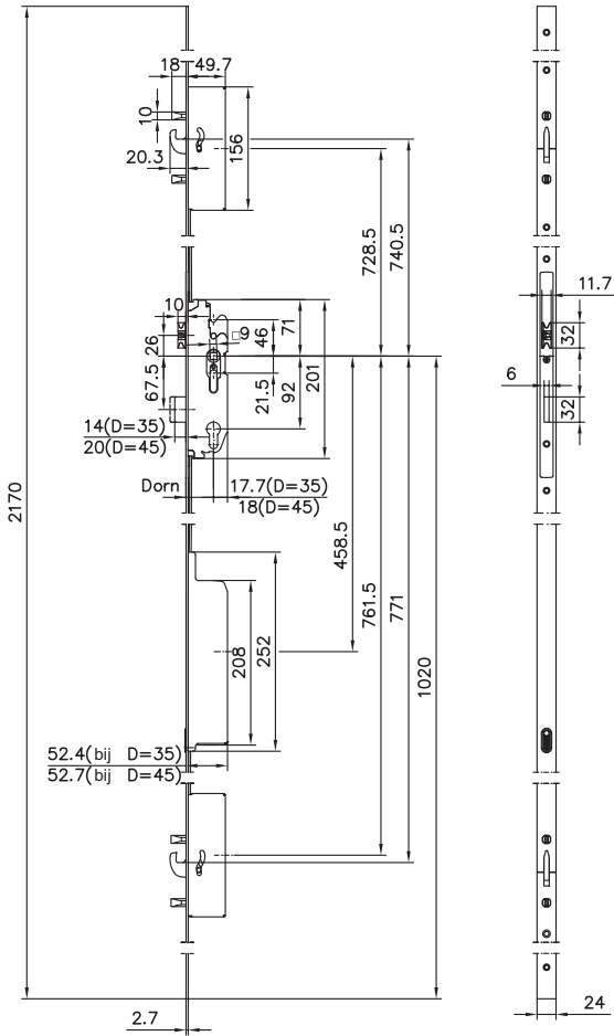
vlakstulp
